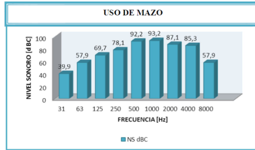
Medición de ruido en banda de octava en ponderación C (impulso)
