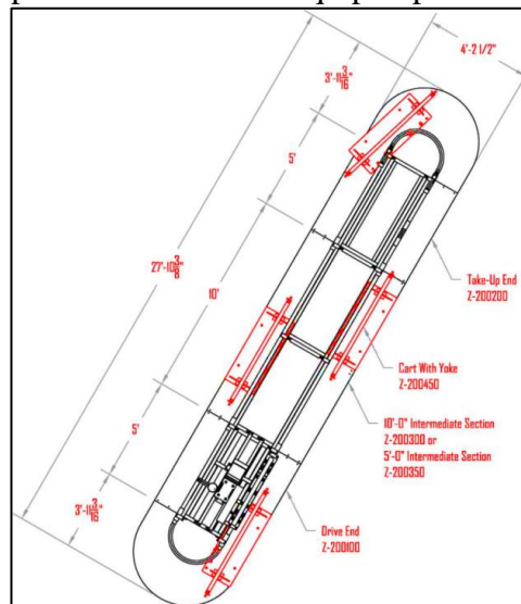
Figura 3. Plano transportador. Fuente: Ensambladora, Los autores
